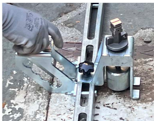
ATTACCO PLUS CON BARRA HOOK
